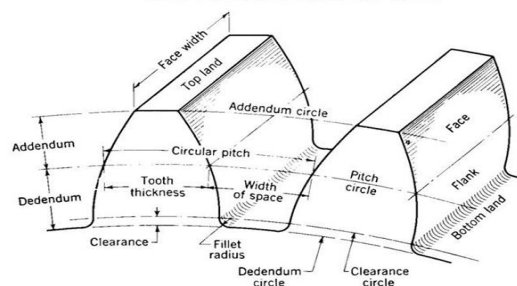
Fig 1. Gear Nomenclature
