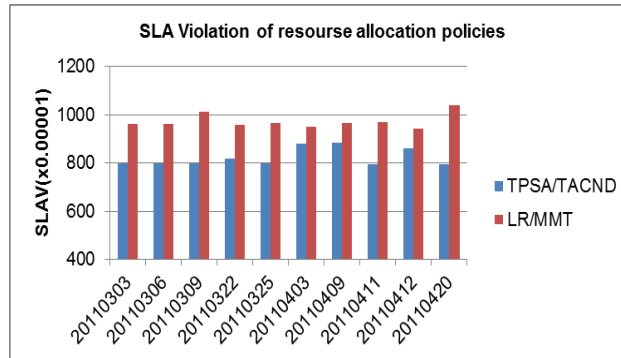
Figure4. SLA Violations
