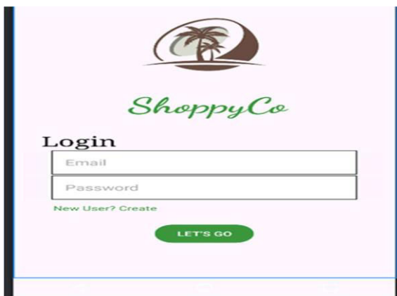
Figure 2 : Login Page
