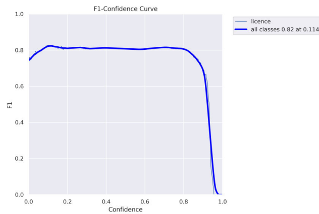
Fig : F1 score of model after testing
