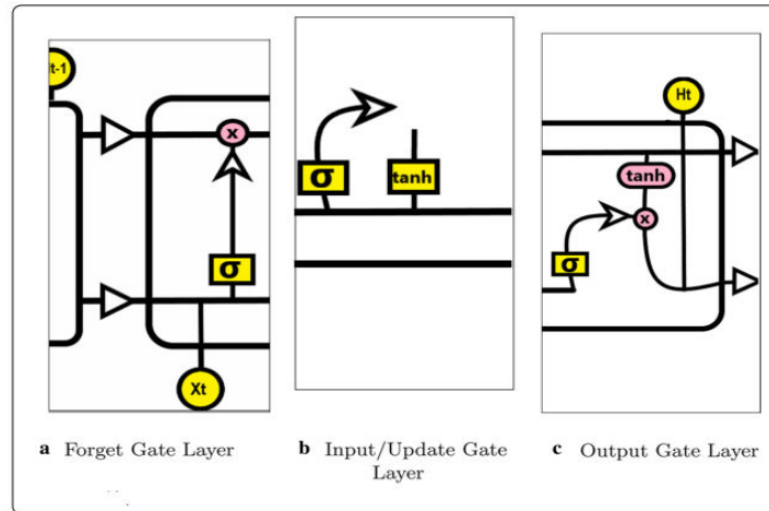
Fig. 4: LSTM Layer
